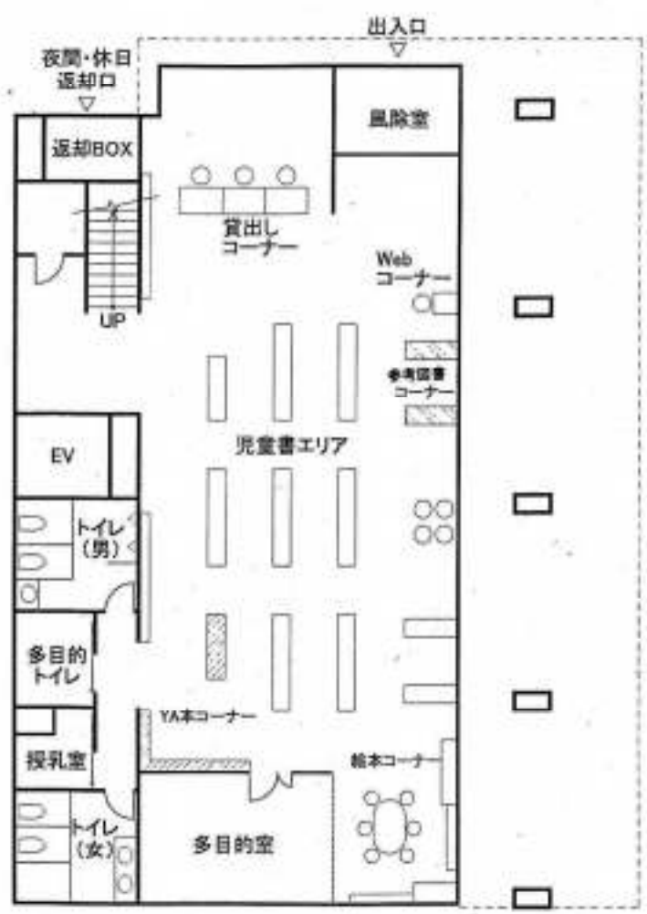
1階平面図
